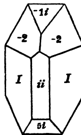
Spinhère.
